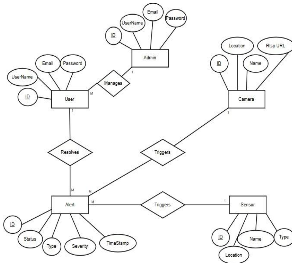
Figure 3.6 : ER Diagram
